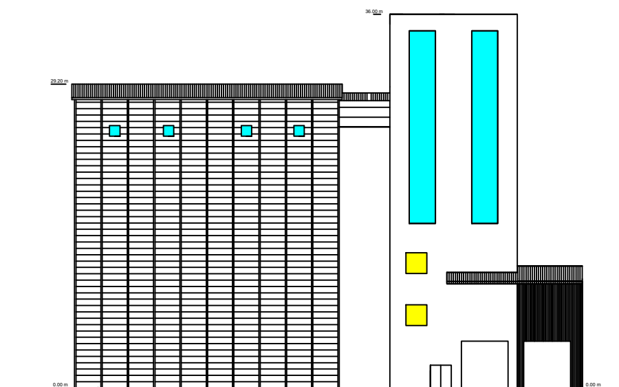
Façade Est
