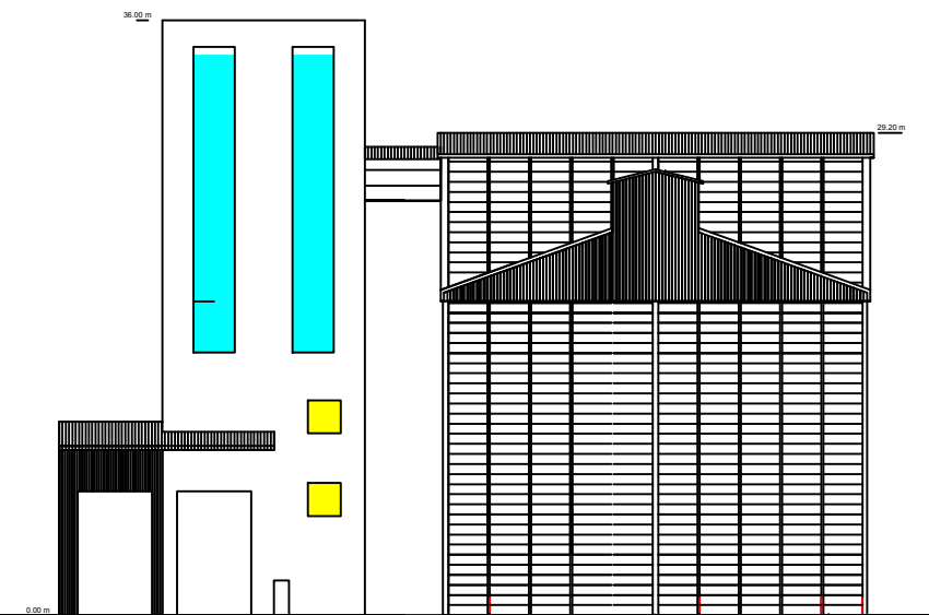
Façade Ouest
