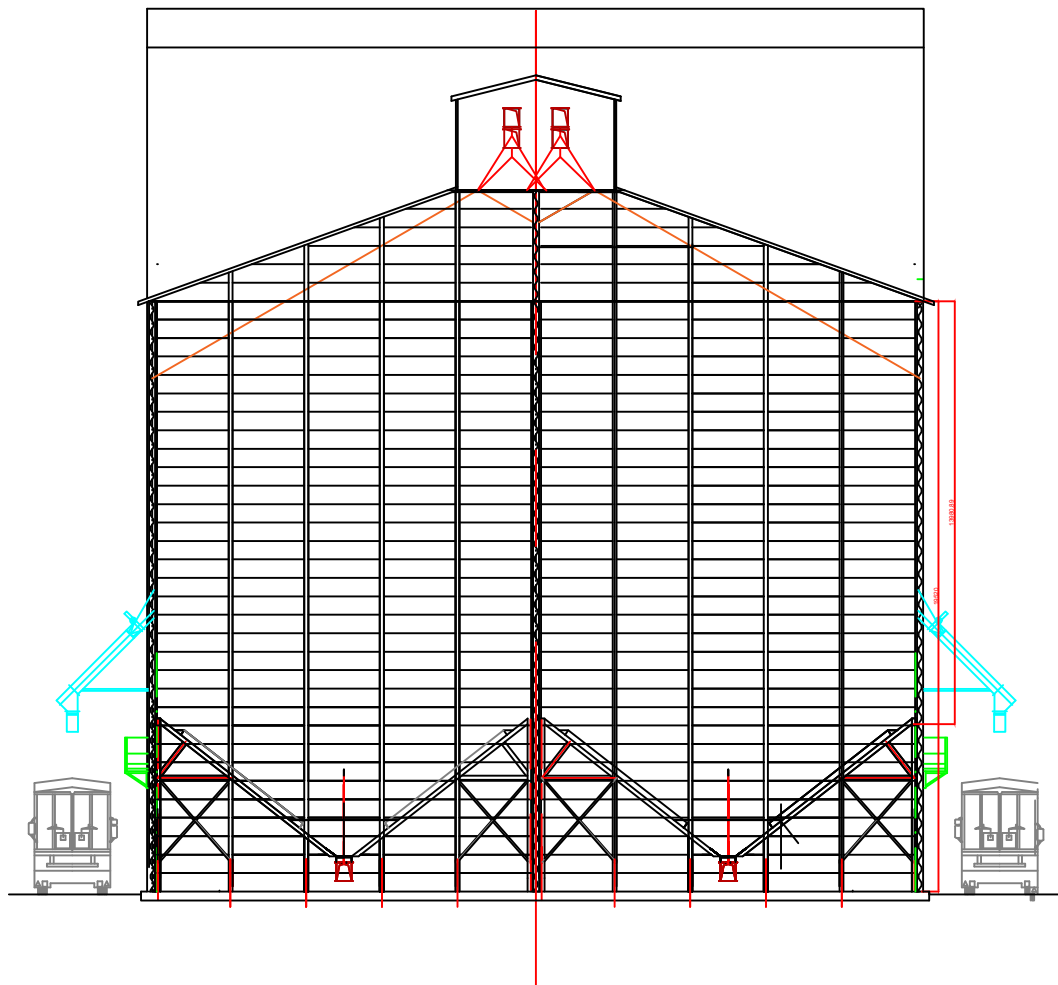
Coupe 1.1
